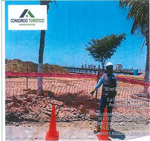
Imagen N°11: Malla de seguridad color anaranjado, cinta color roja y cachacos de concreto.
